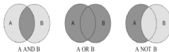
Рис. 2. Диаграммы Венна
